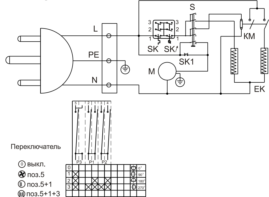
Рис.6. Электрическая схема КЭВ-6С41Е
