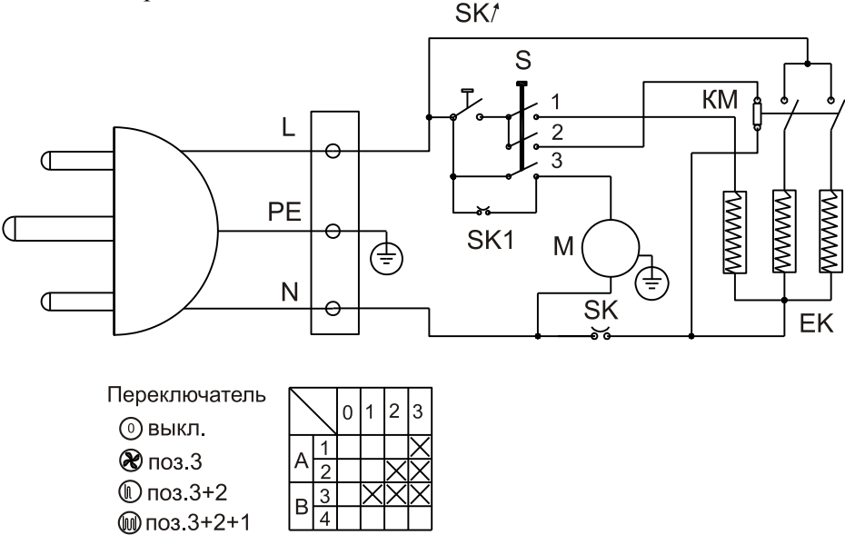
Рис.5. Электрическая схема КЭВ-4С41Е
